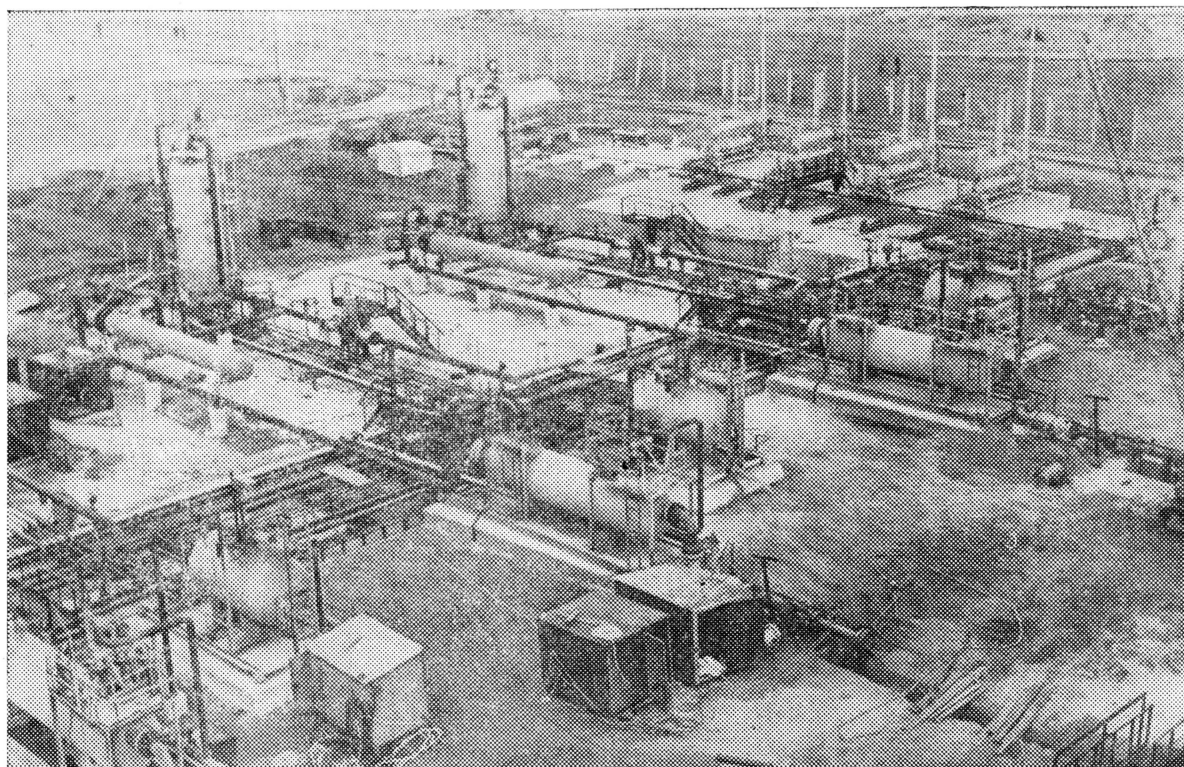
Один из газосборных пунктов
